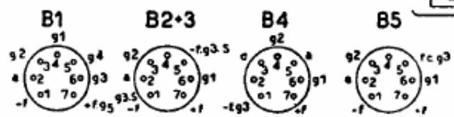
PHILIPS RADIO - Apparecchio portatile a pile-rete mod. LI422 AB. Media frequenza 456 kc. Tre gamme d'onda. Consumo rete 11 W. Consumo batterie 135 V, 12,5 mA; 2,8 V, 150 mA
